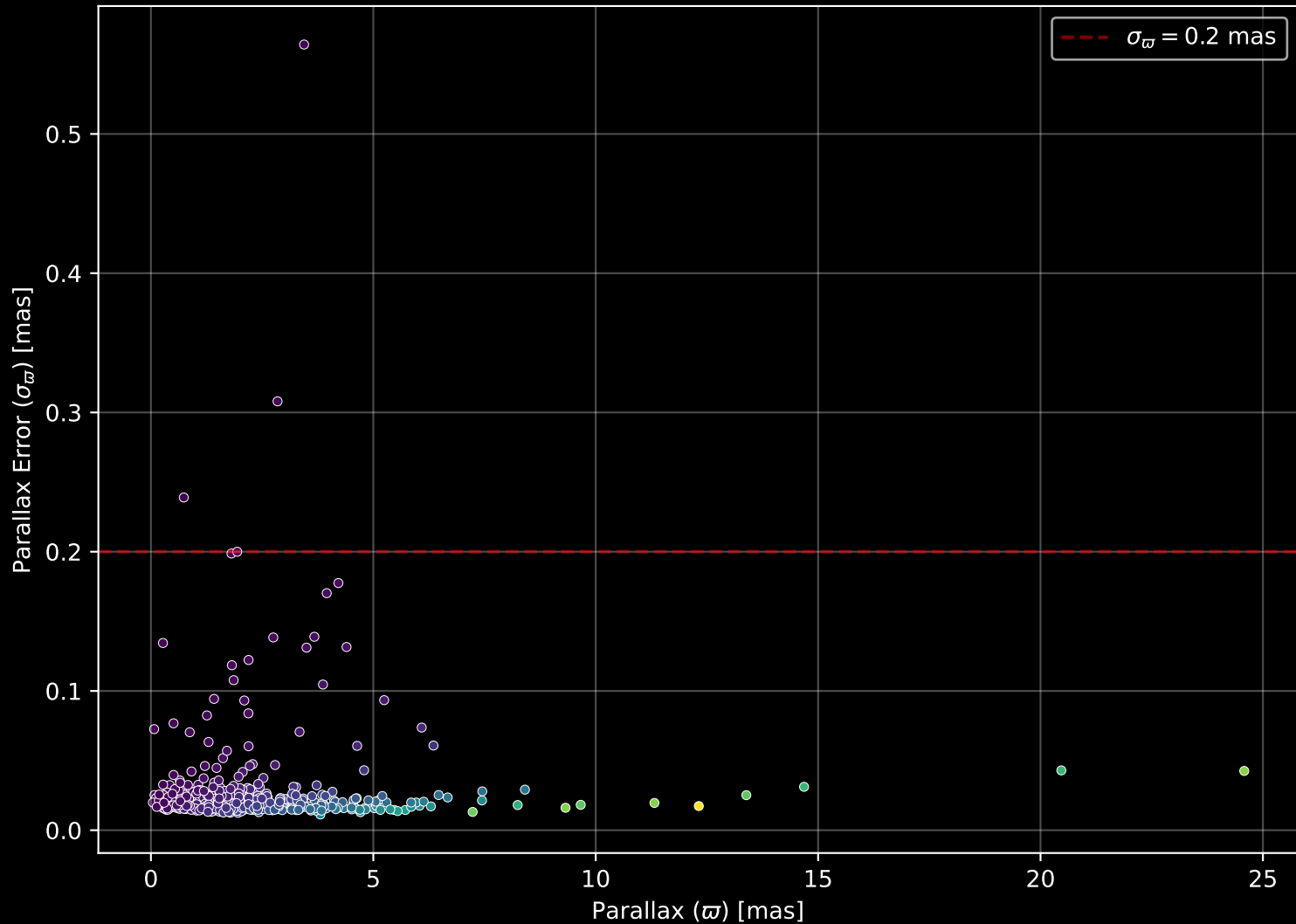
GALAH DR4 Field: [6601] Parallax Quality (n= 462)
