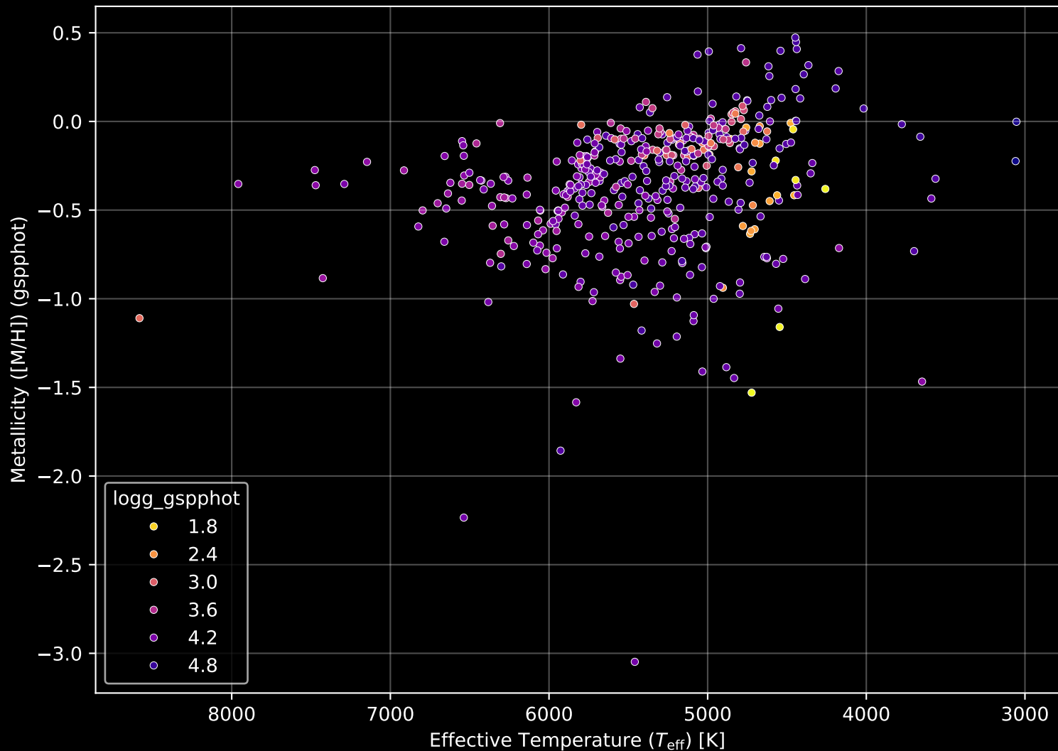
GALAH DR4 Field: [6601] Stellar Population Parameters (n= 462)
