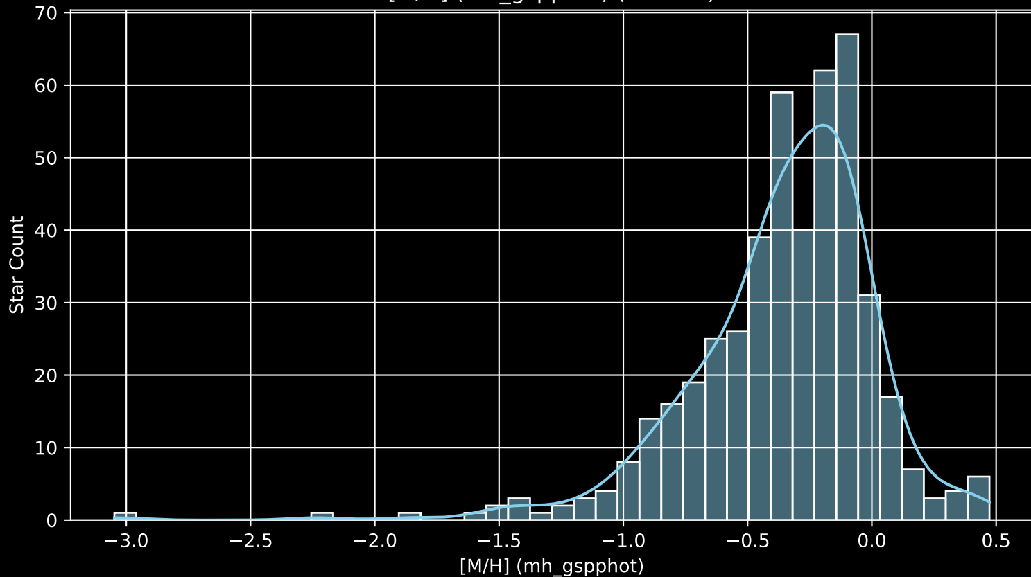
GALAH DR4 Field: [6601] [M/H] (mh_gspphot) (n= 462)
